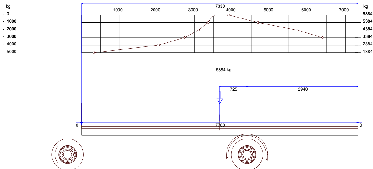
Abb. 1: Lastverteilungsdiagramm Mercedes-Benz Atego 1221L 4x2 mit Standardpritsche
